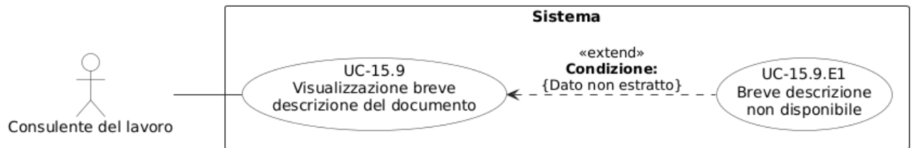
Figura 59: Diagramma del caso d'uso UC-15.9: Visualizzazione breve descrizione del documento
