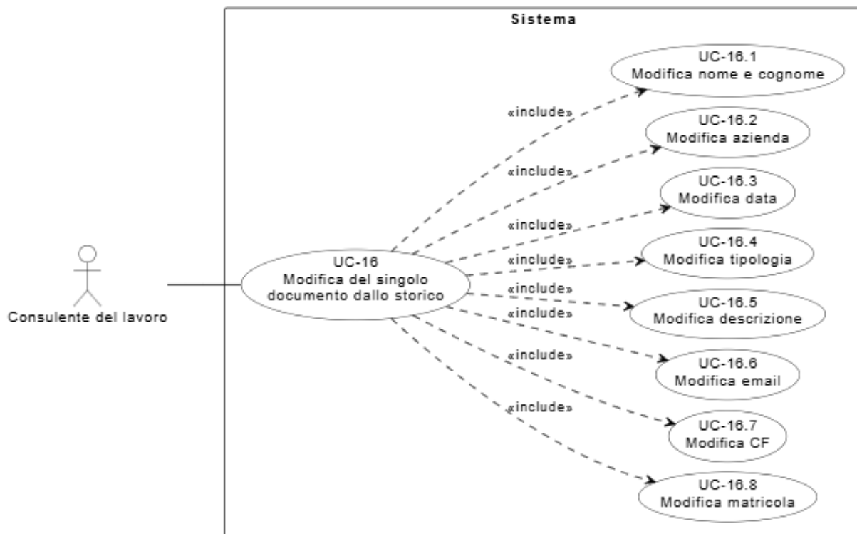
Figura 72: Diagramma del caso d’uso UC-16: Modifica del singolo documento dallo storico
