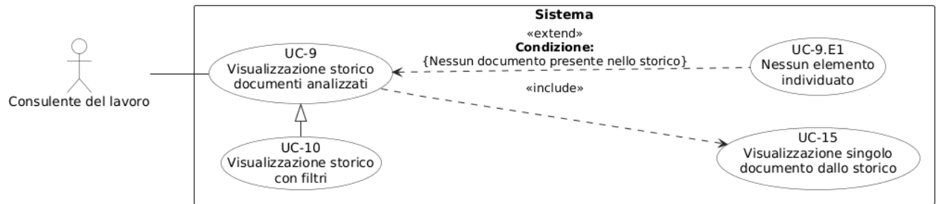
Figura 43: Diagramma del caso d'uso UC-9: Visualizzazione storico documenti analizzati
