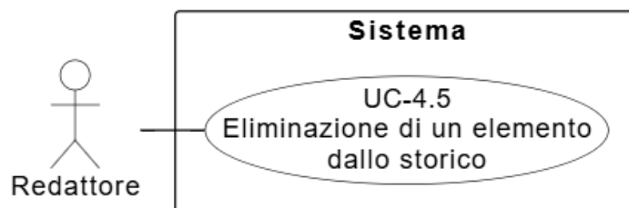
Figura 30: Diagramma del caso d'uso UC-4.5: Elimina elemento dallo storico
