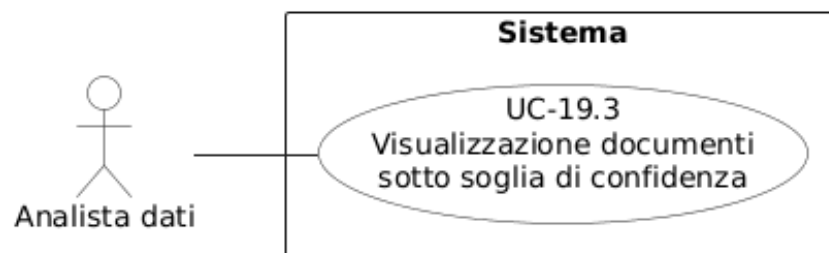
Figura 95: Diagramma del caso d'uso UC-19.3: Visualizzazione documenti sotto soglia di confidenza
