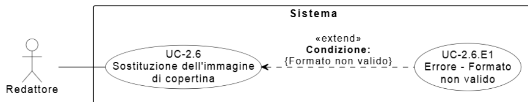
Figura 14: Diagramma del caso d'uso UC-2.6: Sostituisci immagine copertina
