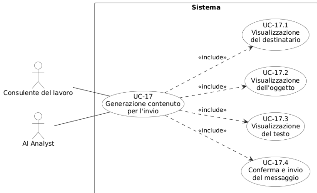
Figura 83: Diagramma del caso d'uso UC-17: Generazione contenuto per l'invio
