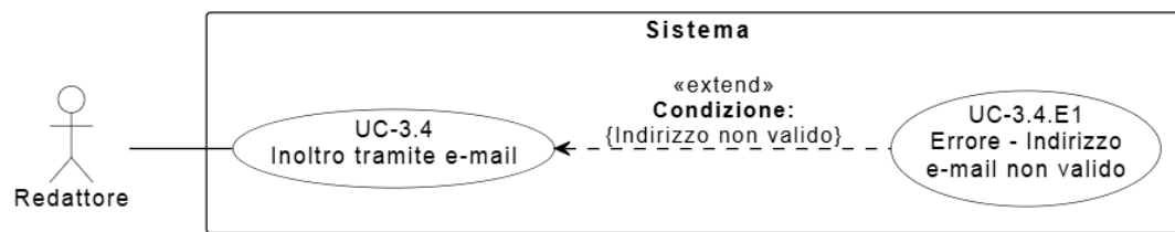
Figura 21: Diagramma del caso d’uso UC-3.4: Inoltra documento via e-mail
