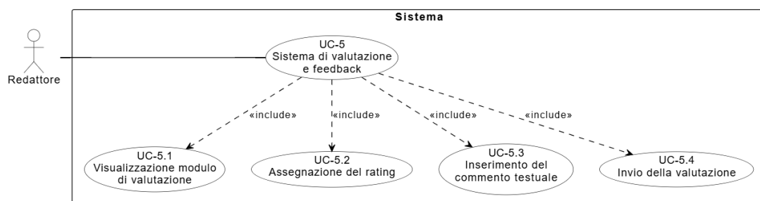
Figura 31: Diagramma del caso d'uso UC-5: Valuta bozza generata
