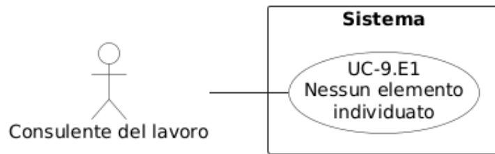
Figura 44: Diagramma del caso d'uso UC-9.E1: Nessun elemento individuato
