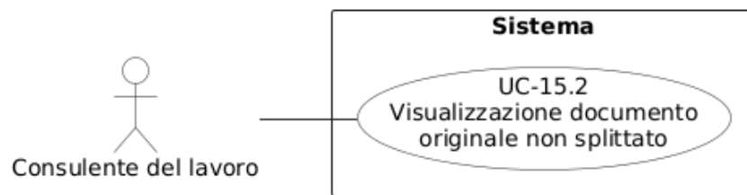
Figura 52: Diagramma del caso d'uso UC-15.2: Visualizzazione documento originale non splittato
