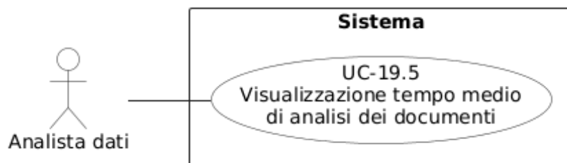
Figura 97: Diagramma del caso d'uso UC-19.5: Visualizzazione tempo medio di analisi dei documenti
