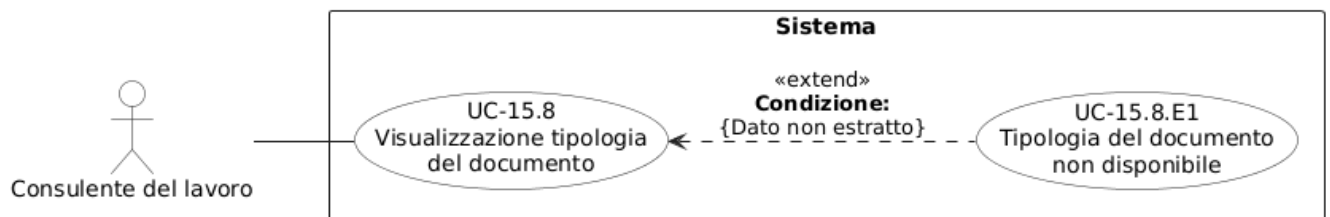
Figura 58: Diagramma del caso d'uso UC-15.8: Visualizzazione tipologia del documento
