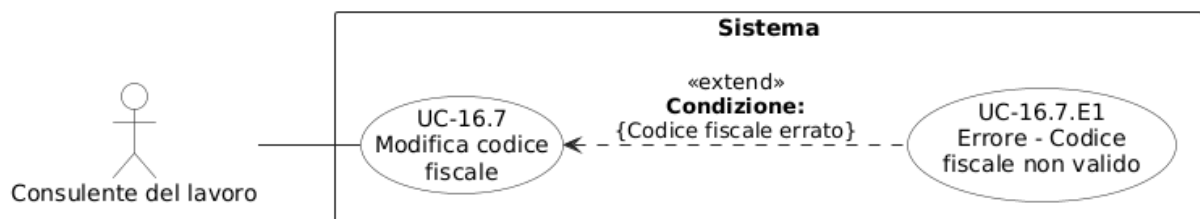
Figura 79: Diagramma del caso d'uso UC-16.7: Modifica codice fiscale
