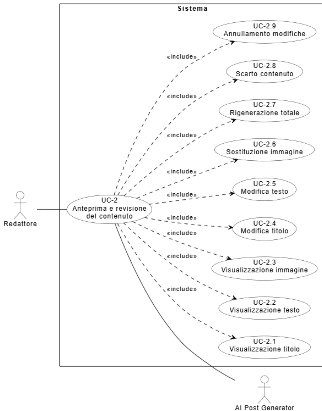
Figura 8: Diagramma del caso d'uso UC-2: Visualizzazione anteprima bozza generata
