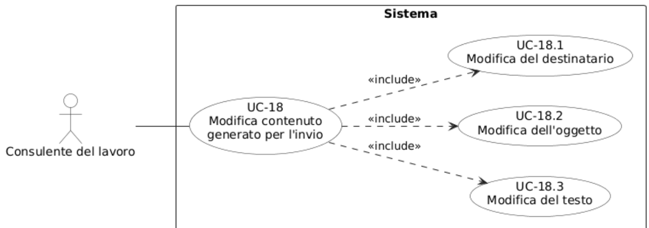
Figura 88: Diagramma del caso d'uso UC-18: Modifica contenuto generato per l'invio
